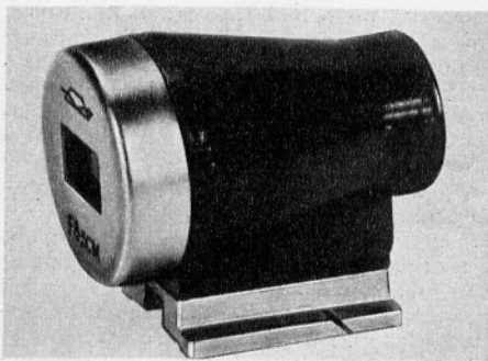
Фото 1. Видоискатель ВИ для объектива с фокусным расстоянием 85 мм к фотоаппаратам с кадром 24x36 мм
